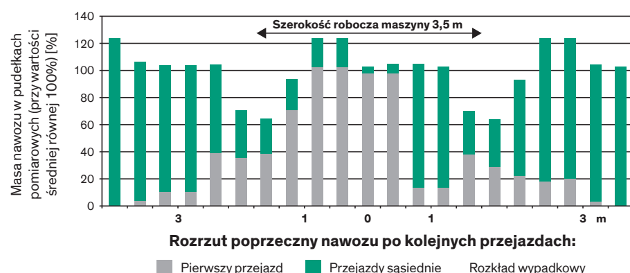
Wyk. 1. Rozkład poprzeczny obornika rozrzućnikiem Jeantil EP 2060 Epandor 2 z adapterem dwubębnowym poziomym, przy szerokości roboczej 3,5 m [Frick i in. 2001, Ausbringtechnik Abfalldünger und Laufstallmist].
