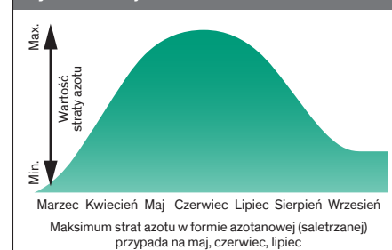
Rys. 2. Potencjalna strata azotu.
