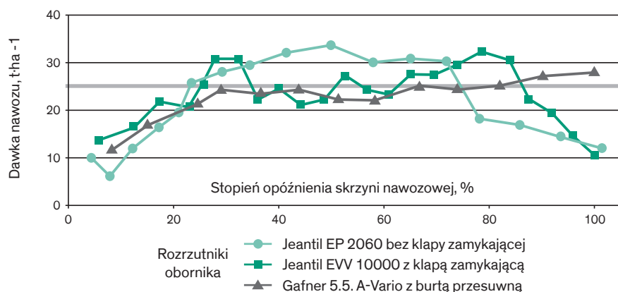
Wyk. 2. Dokładność rozkładu wzdłużnego kompostu przy założonej dawce 25 t·ha -1 , rozrzućanym rozrzućnikami Jeantil EP 2060 (bez klapy zamykającej), Jeantil EVV 10000 (z klapy zamykającą) i Gafner 5.5 - Vario (z burtą przesuwającą) [Źródło: Frick i in. 2001, Ausbringtechnik Abfalldünger und Laufstallmist].
